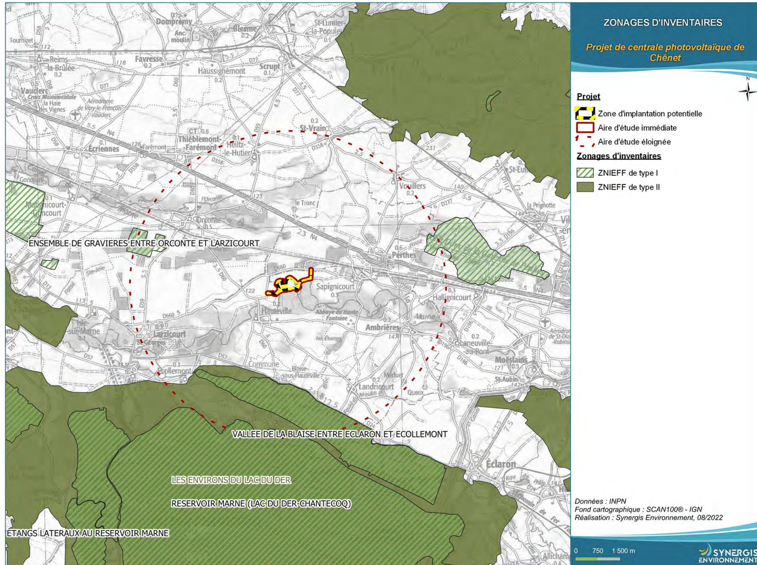
Figure 62 : Zonages d'inventaires
