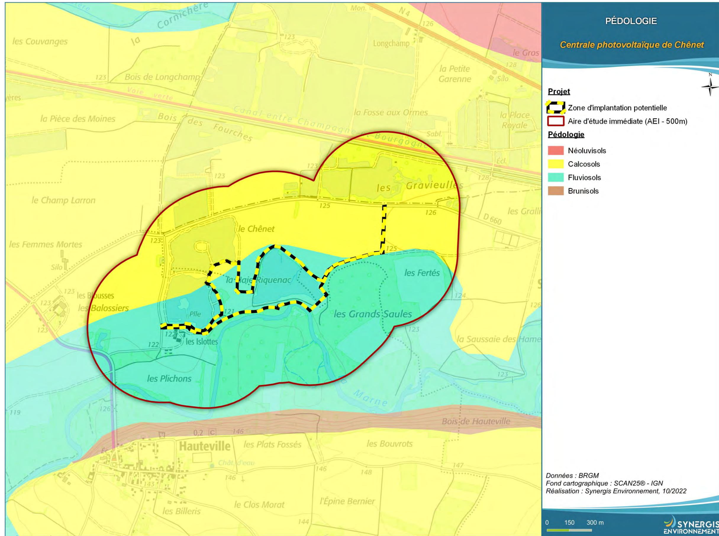
Figure 36 : Pédologie
