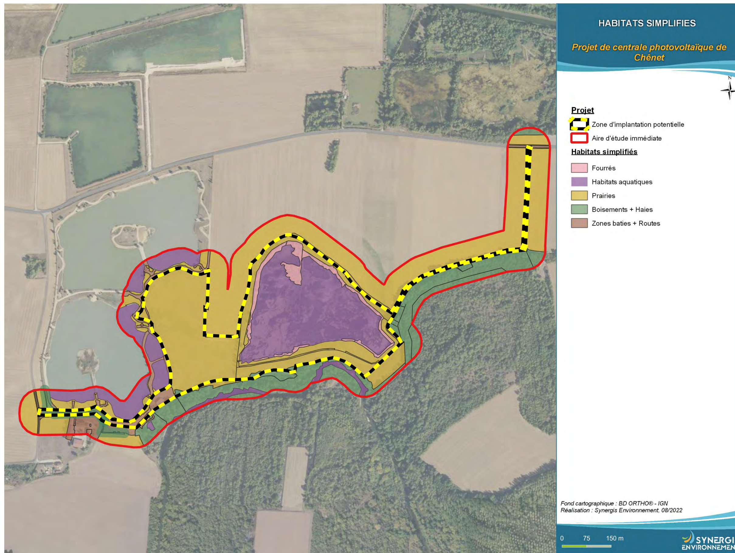
Figure 66 : Habitats simplifiés
