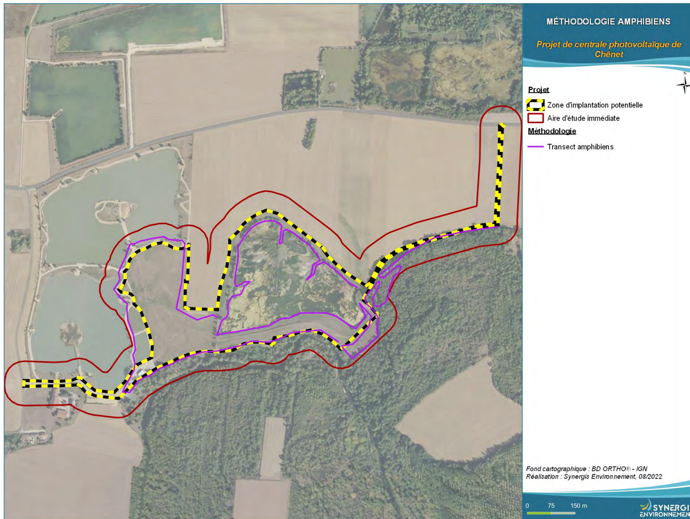
Figure 19 : Méthodologie amphibiens
