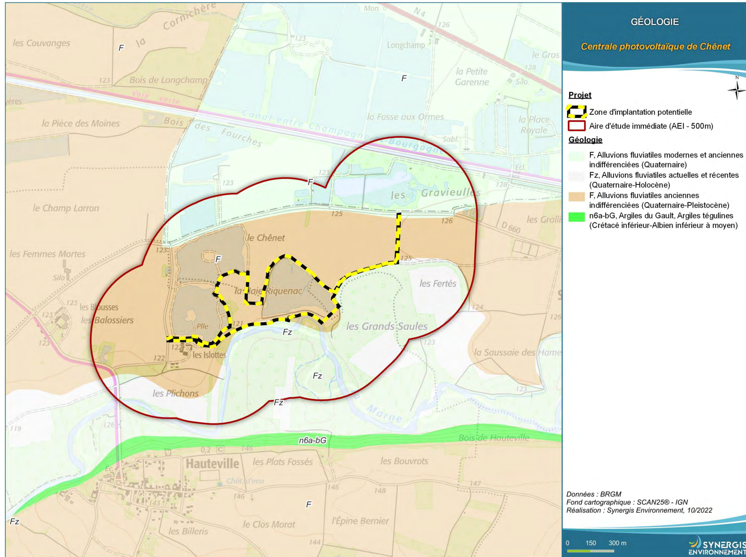
Figure 35 : Géologie
