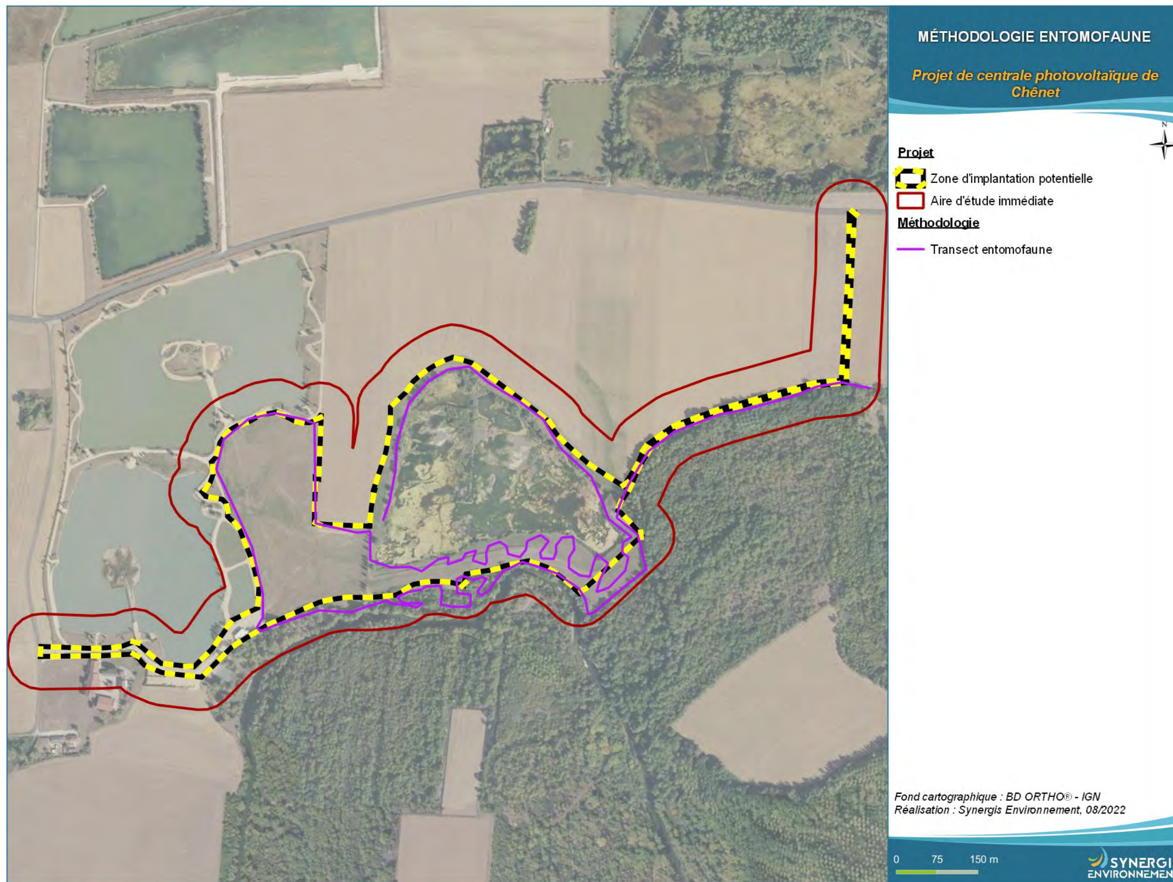
Figure 21 : Méthodologie entomofaune
