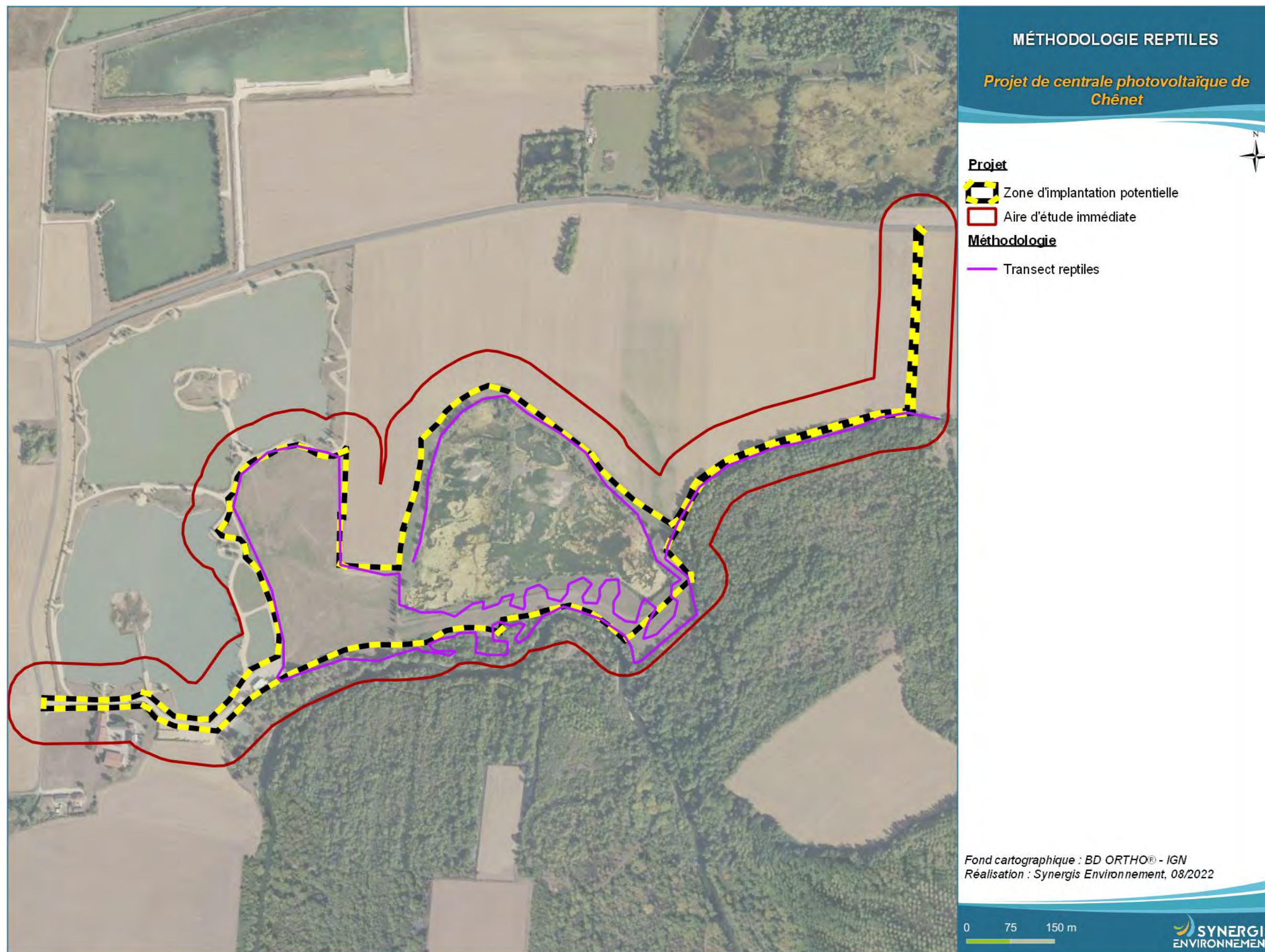
Figure 20 : Méthodologie reptile
