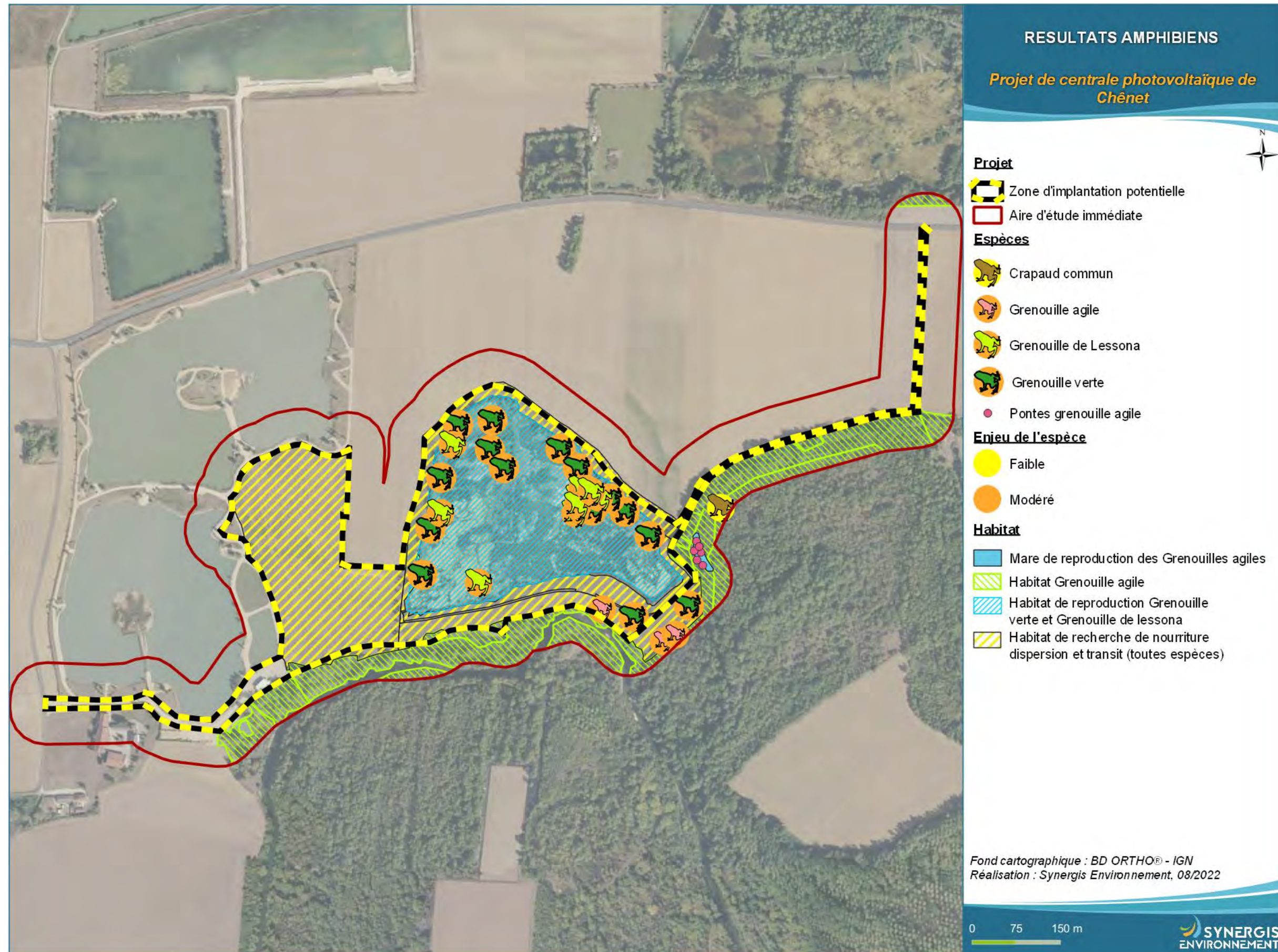
Figure 86 : Résultats amphibiens
